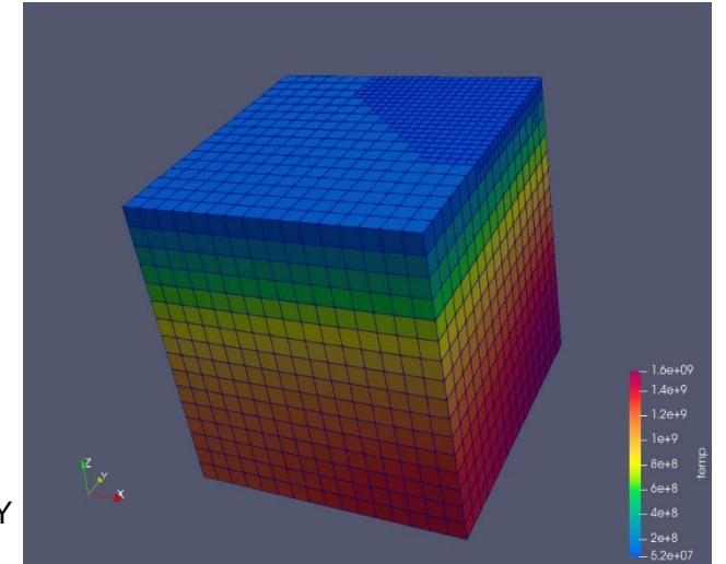
pHEAT-3D: 熱伝導アプリケーション 直方体の場合はX-Y-Z 分割割り当て
